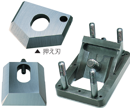
▲ 切刃
